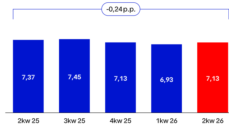
Wskaźnik dźwigni [%]
